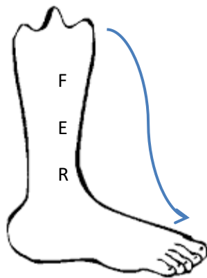
Fer / argile
